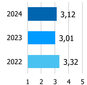
Keskiarvo (asteikko 1-5)
