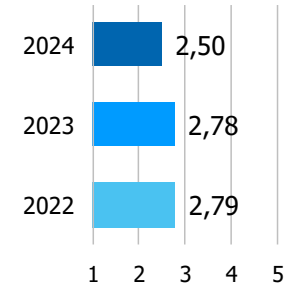
Keskiarvo (asteikko 1-5)
