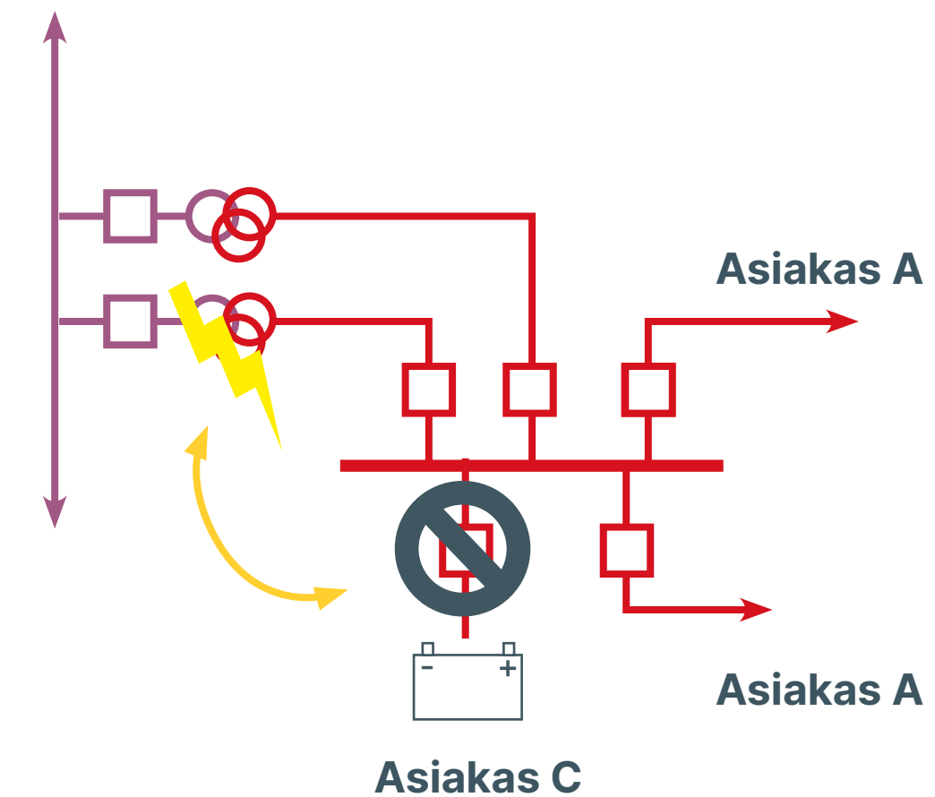
Toisen muuntajan vikaantuminen: Joustavalla liittymällä oleva asiakas C irtikytkeytyy verkosta
